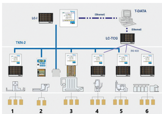
Slika 6: Prikaz kontrolnega sistema izdelovalca Trützschler: 1 – rahljalnik bal (potujoči odzvalnik), 2 – rahljalnik bal s poševnim iglastim trakom, 3 – mešalna komora, 4 – vertikalni rahljalnik/čistilnik, 5 – mikalnik s pokrovčki, 6 – valjčni raztezalnik [6]
