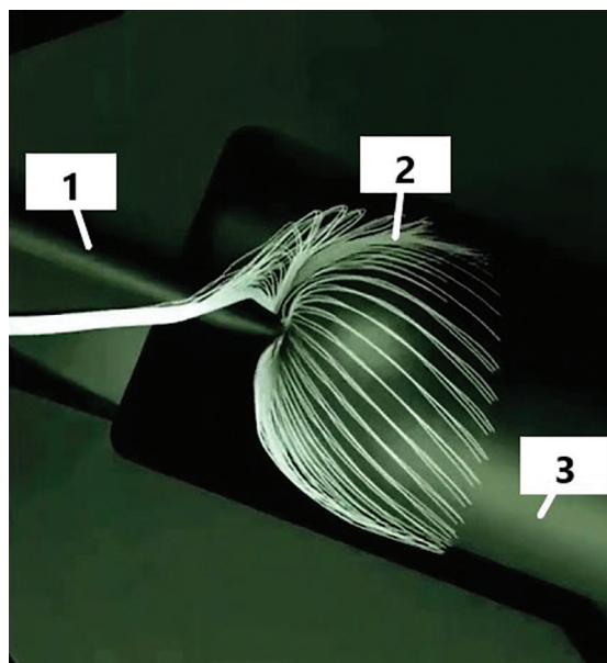
Slika 31: Prikaz igle za preusmerjanje vlaken k votlemu vretenu in pahljače vlaken, ki se ustvari na predilniku VORTEX 870 EX: 1 – igla za preusmerjanje vlaken, 2 – pahljača vlaken, 3 – votlo vreteno [14]
