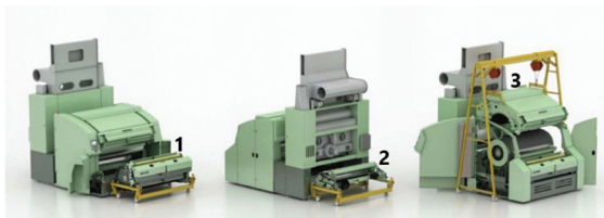
Slika 10: Prikaz preproste menjave posameznih delov mikalnika C77: 1 – prikaz menjave snemalnega valja, 2 – prikaz menjave dovajalnega in rahljalnega valja, 3 – prikaz menjave pokrovčkov [5]
